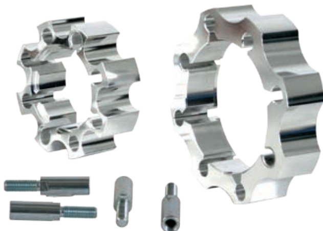
WHEELS SPACERS / 45 mm DISTANZIALI ALLARGATORI RUOTE / 45 mm
